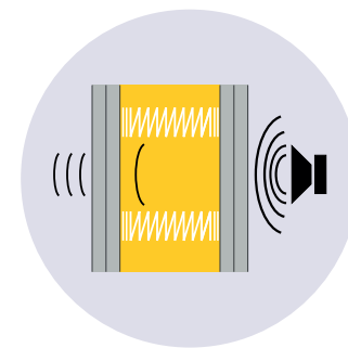
Gušenje zvuka montažnog pregradnog zida po principu: masa – opruga – masa
